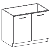
alsó szekrény 2 ajtós 80 D 2F BB 800x820x520 (szélesség/magasság/mélyiség)
