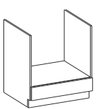
sütő beépítés 60 D GAZ BB 600x820x520 (szélesség/magasság/mélyiség)
