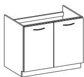
mosogatószekrény 2 ajtós 80 ZL 2F BB 800x820x520 (szélesség/magasság/mélyiség)
